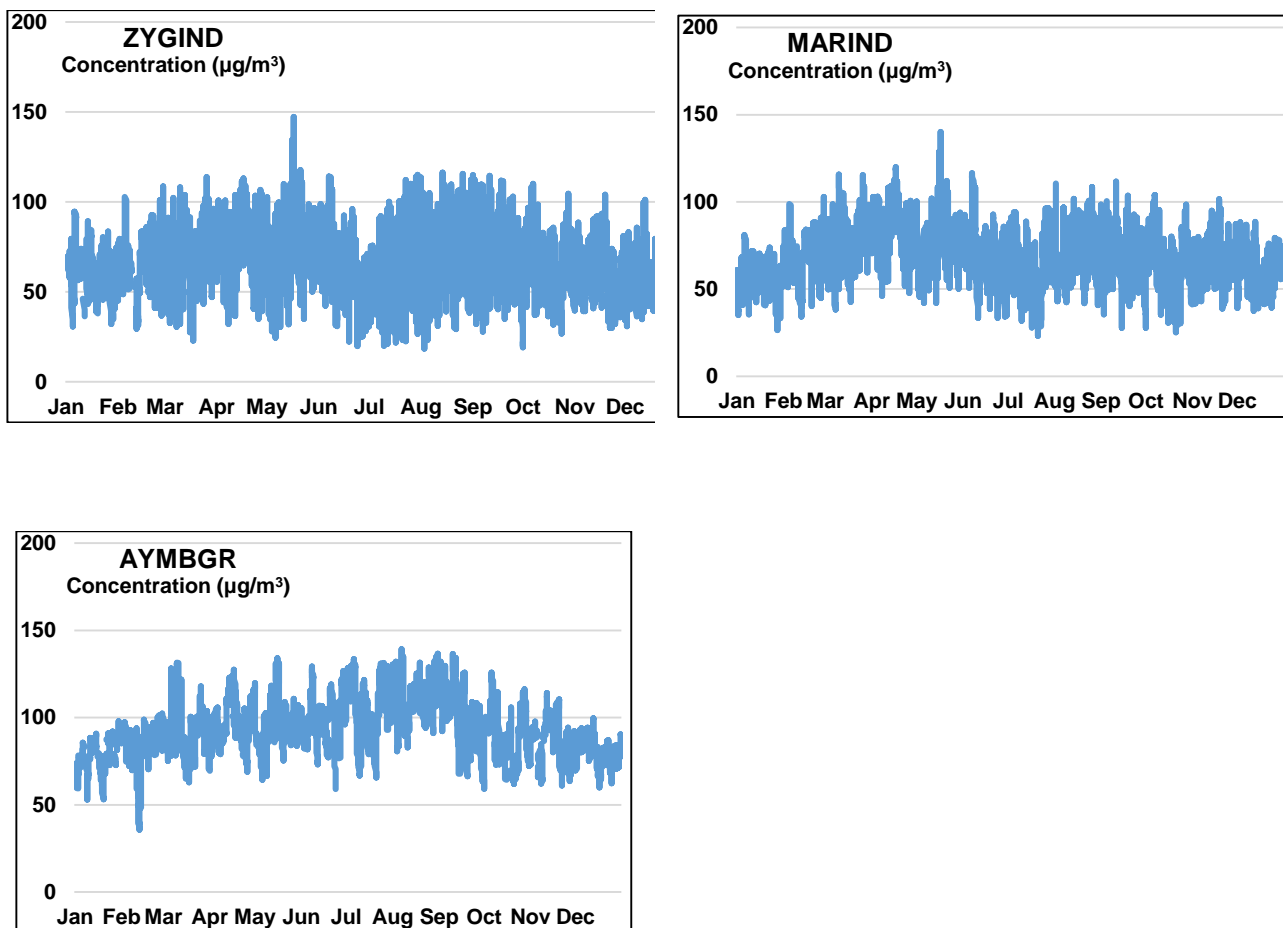
Σχήμα 8: Μέσες 8-ωρες τιμές όζοντος ( O_3 ) στους Σταθμούς Παρακολούθησης Ποιότητας Αέρα για το έτος 2020 (Μέγιστος ημερήσιος μέσος όρος οκταώρου – Τιμή Στόχος: 120 \mu\text{g}/\text{m}^3 ).
