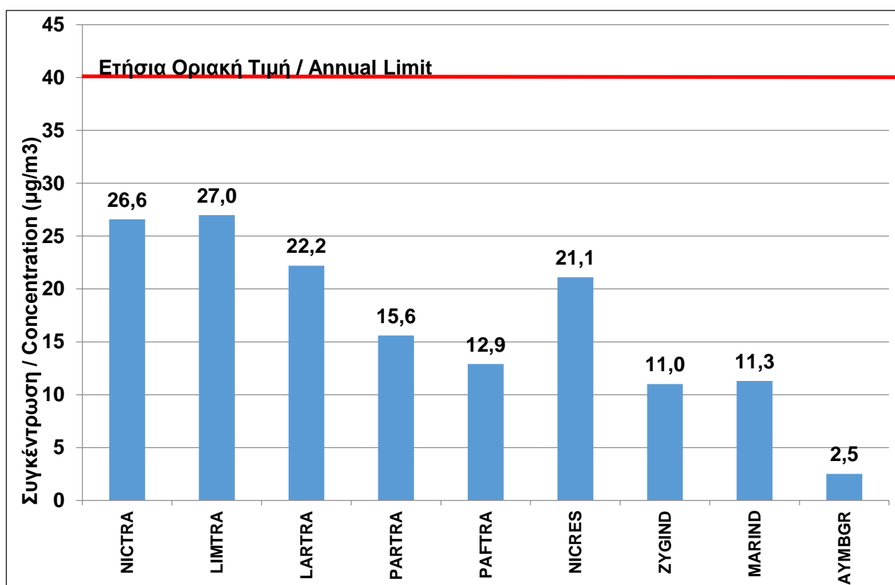
Σχήμα 4: Ετήσιοι μέσοι όροι \text{NO}_2 στους Σταθμούς Παρακολούθησης Ποιότητας Αέρα για το έτος 2020.
