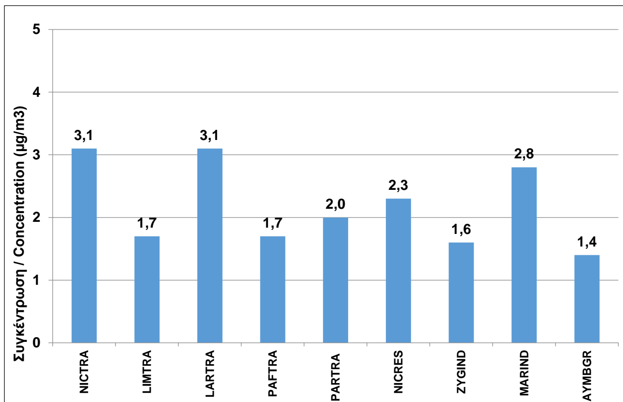
Σχήμα 6: Ετήσιοι μέσοι όροι \text{SO}_2 στους Σταθμούς Παρακολούθησης Ποιότητας Αέρα για το έτος 2020. Figure 6: \text{SO}_2 annual mean concentration in Air Quality Monitoring Stations for the year 2020.
