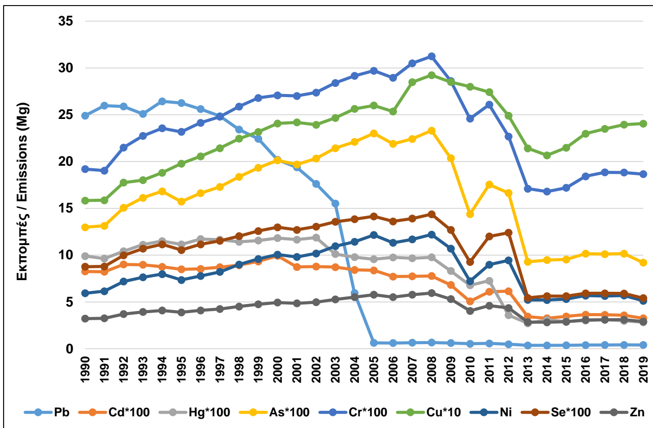
Σχήμα 21: Τάσεις εκπομπών για τα βαρέα μέταλλα για την περίοδο 1990-2019. Figure 21: Emission trends for heavy metals for the period 1990-2019.
