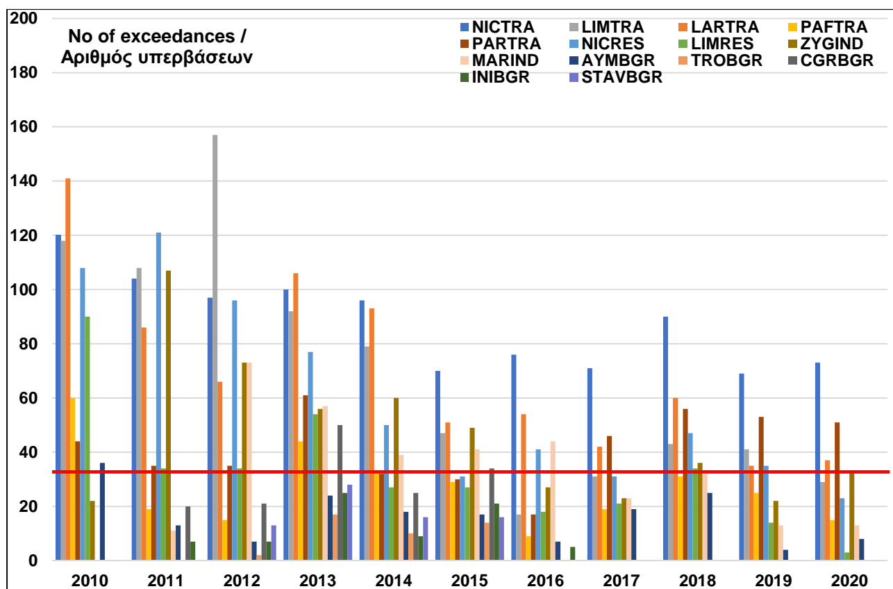
Σχήμα 12: Αριθμός υπερβάσεων ανά έτος της ημερήσιας οριακής τιμής ΑΣ 10 στους Σταθμούς Παρακολούθησης Ποιότητας Αέρα για την περίοδο 2010-2020 (Αριθμός επιτρεπτών υπερβάσεων: 35).
