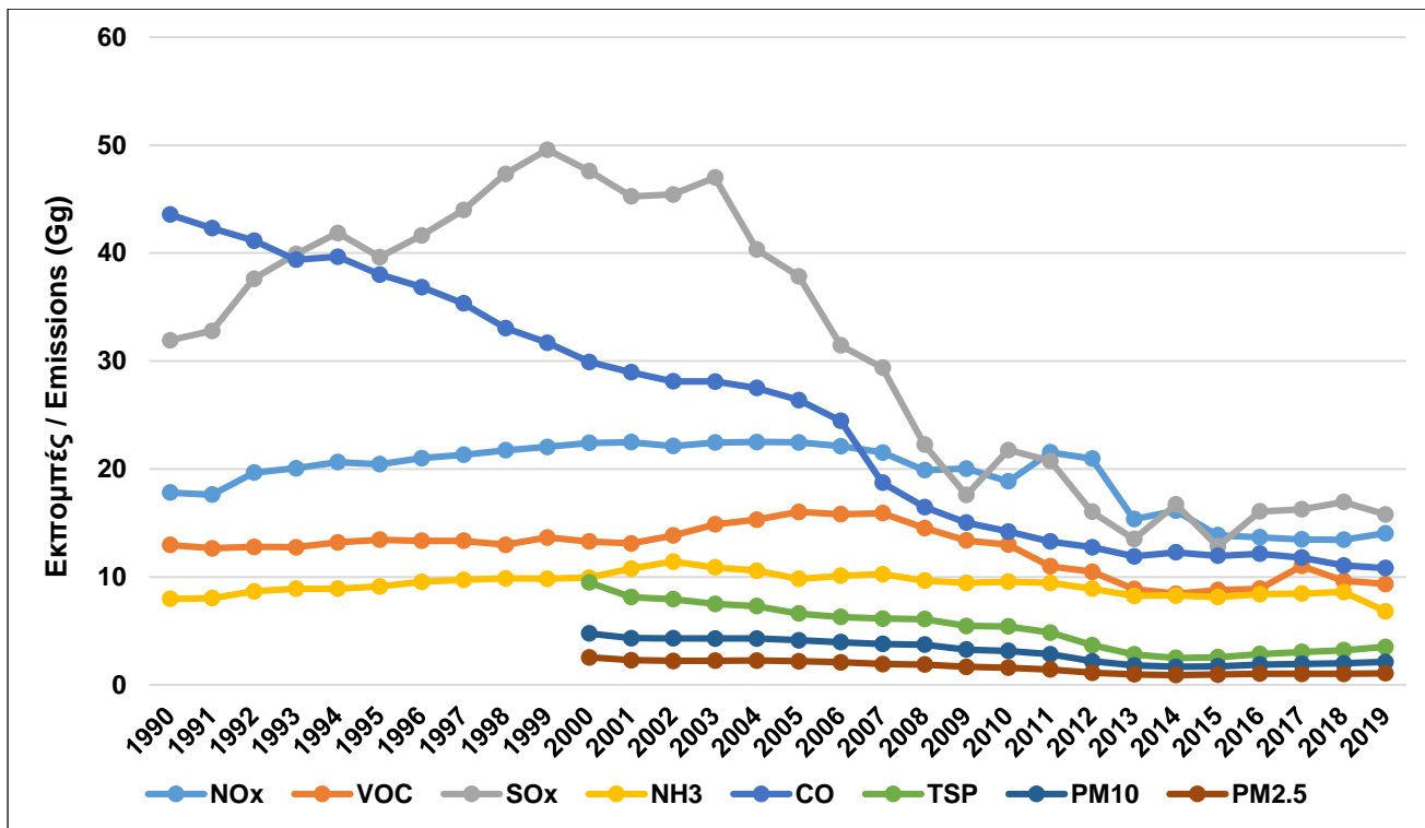
Σχήμα 20: Τάσεις εκπομπών για τους κύριους ρύπους και τα σωματίδια για την περίοδο 1990-2019. Figure 20: Emission trends for main pollutants and particulates for the period 1990-2019.
