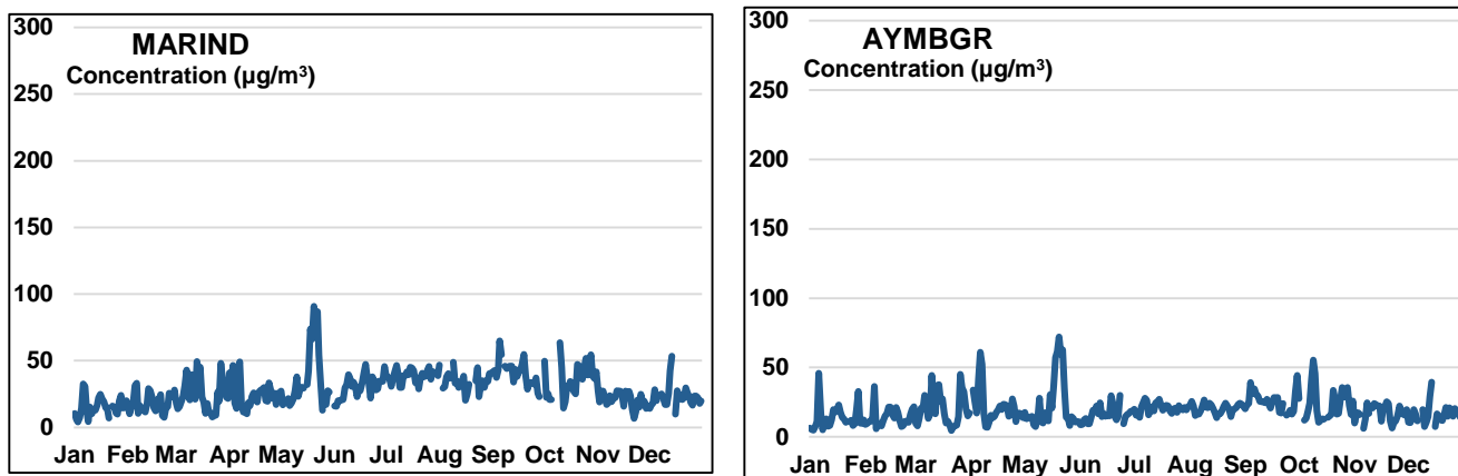
Σχήμα 14: Ημερήσια συγκέντρωση Αιωρούμενων Σωματιδίων με αεροδυναμική διάμετρο 10 µm (ΑΣ 10 ) στους Σταθμούς Παρακολούθησης Ποιότητας Αέρα για το έτος 2020 (Ημερήσια οριακή τιμή: 50 µg/m 3 ).
