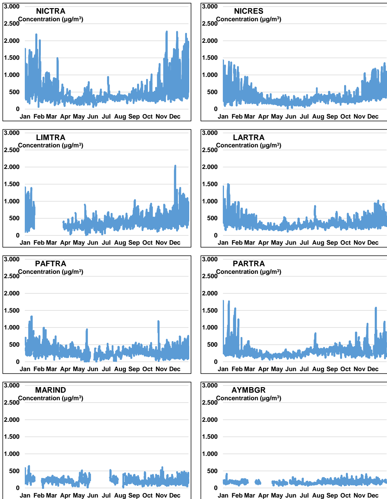
Σχήμα 10: Μέσες 8-ώρες τιμές μονοξειδίου του άνθρακα (CO) στους Σταθμούς Παρακολούθησης Ποιότητας Αέρα για το έτος 2020 (Οριακή Τιμή μέγιστου ημερήσιου μέσου όρου οκταώρου: 10.000 \mu\text{g}/\text{m}^3 ).
