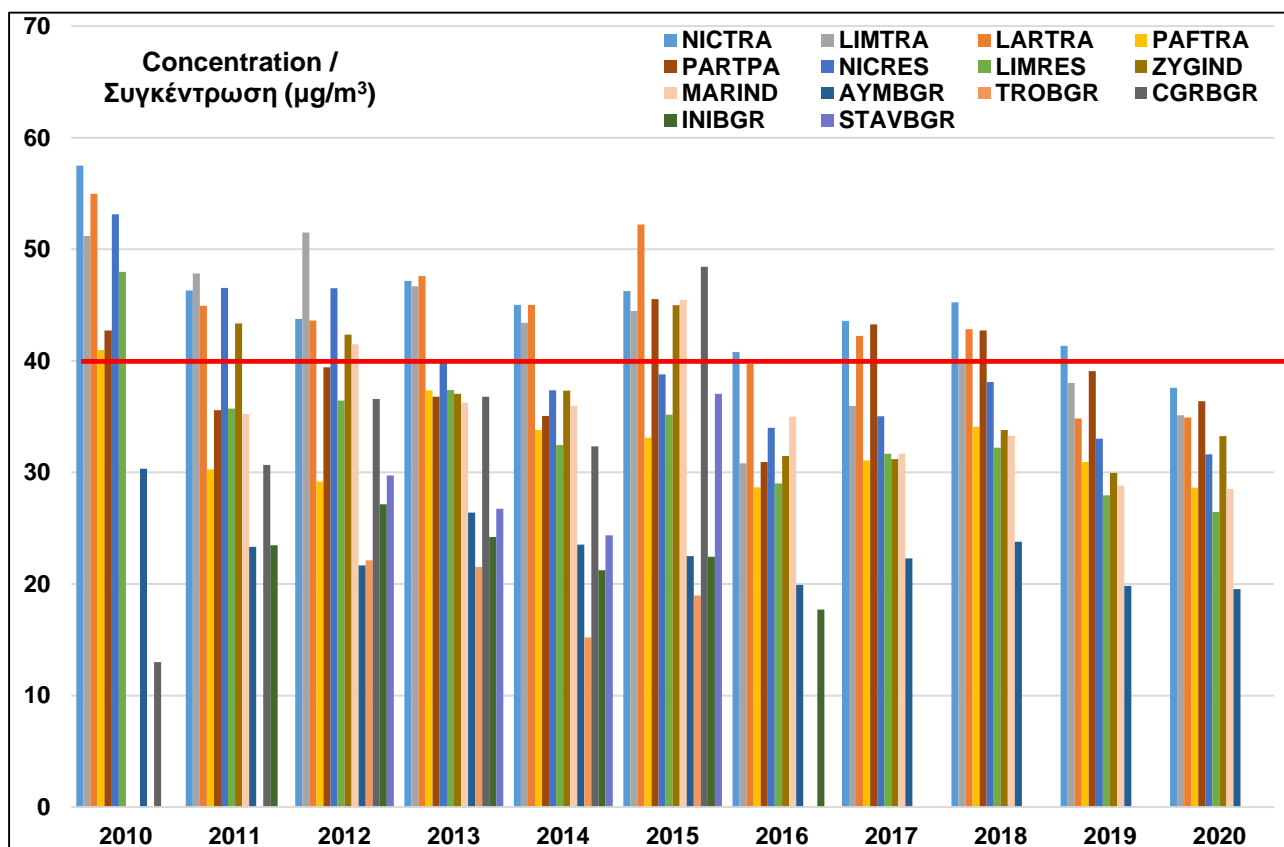
Σχήμα 11: Ετήσιοι μέσοι όροι ΑΣ 10 στους Σταθμούς Παρακολούθησης Ποιότητας Αέρα για την περίοδο 2010-2020 (Ετήσια οριακή τιμή: 40 µg/m 3 ).
