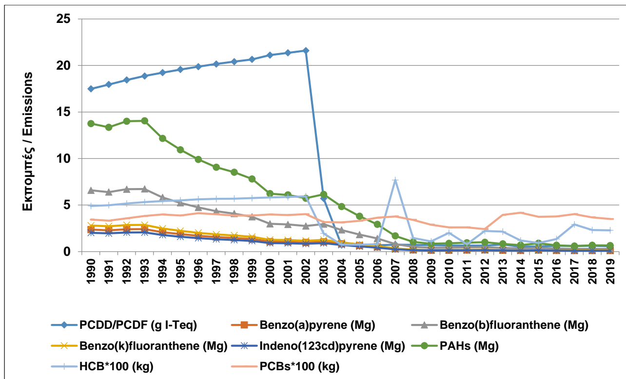
Σχήμα 22: Τάσεις εκπομπών για τους Έμμοιους Οργανικούς Ρύπους για την περίοδο 1990-2019.
