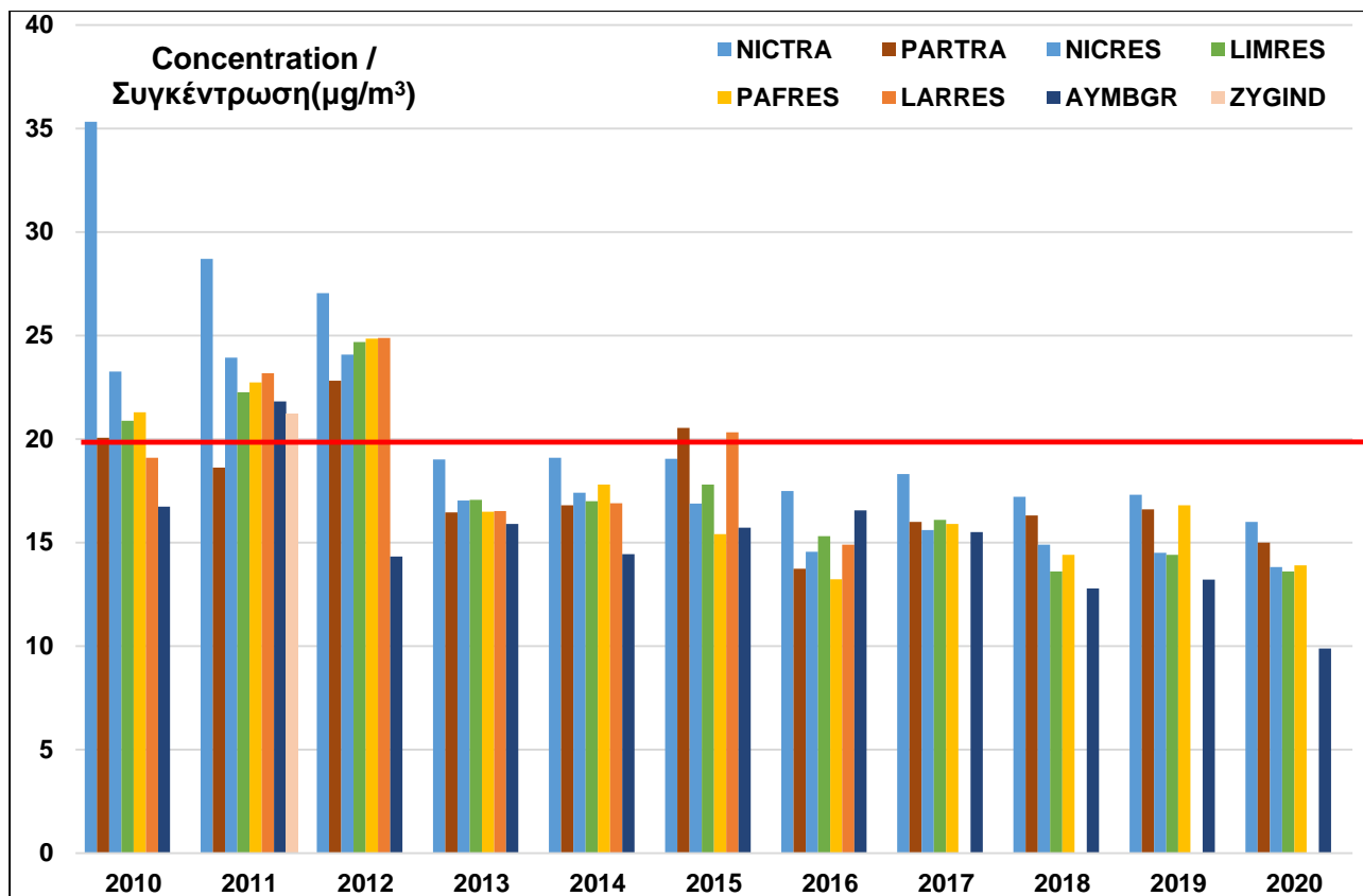
Σχήμα 13: Ετήσιοι μέσοι όροι ΑΣ 2,5 στους Σταθμούς Παρακολούθησης Ποιότητας Αέρα για την περίοδο 2010-2020 (Ετήσια οριακή τιμή: 20 µg/m 3 ).
