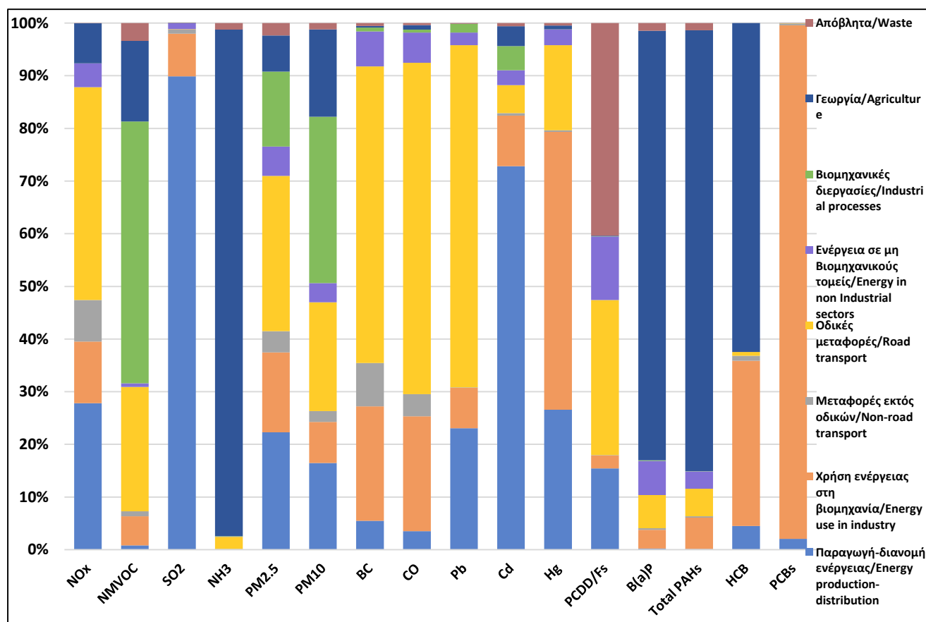
Σχήμα 19: Κατανομή (%) των συνολικών εκπομπών ανά κατηγορία για το 2019. Figure 19: Share (%) of national total emissions, by sector group in 2019.
